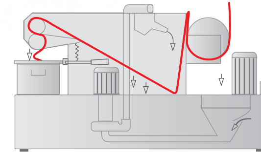
Hidrostatik filtre sistemleri (Knoll, BMF)
