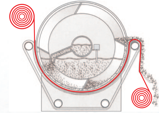
Tambur filtre sistemleri
